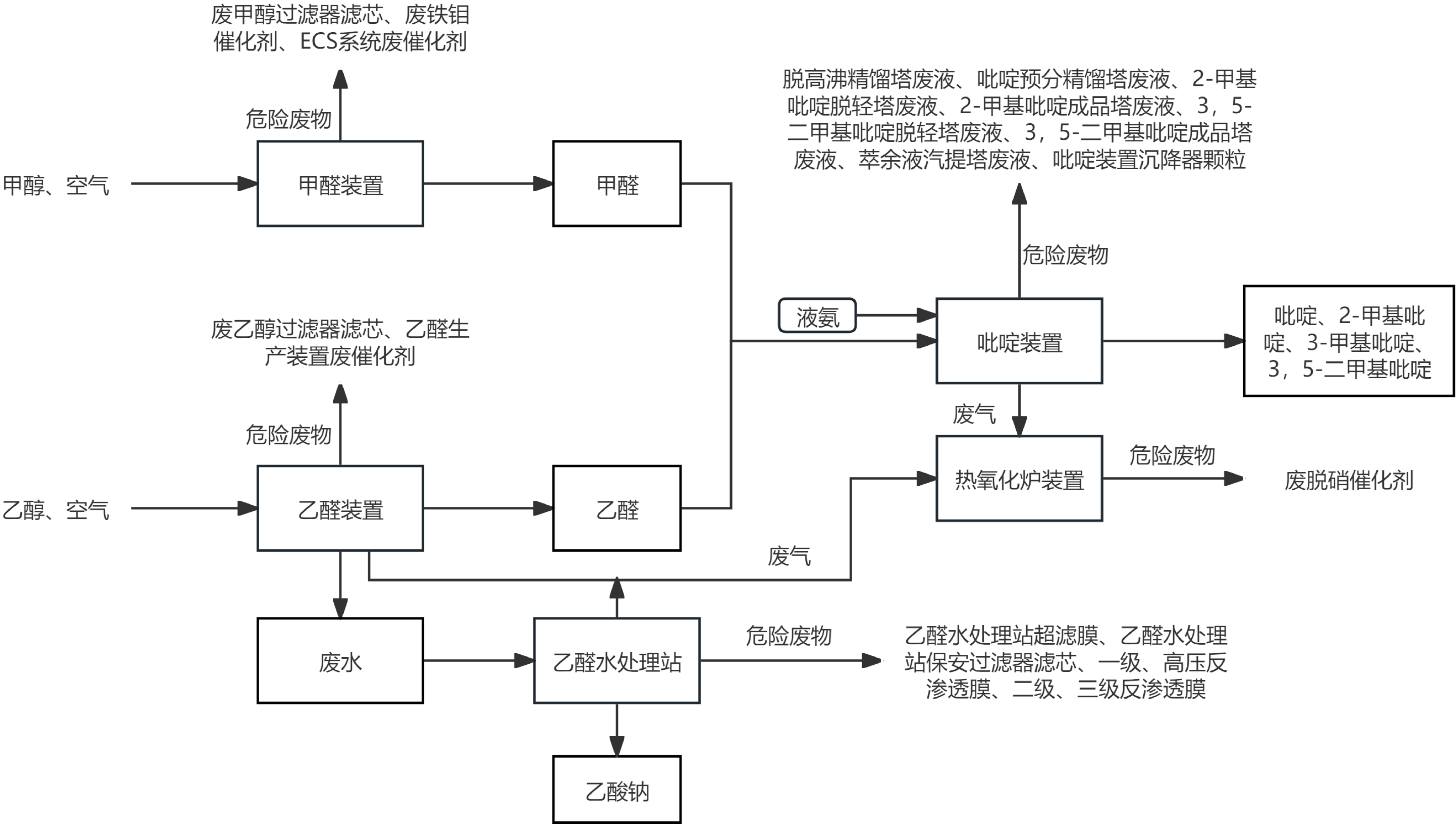
危险废物产生环节图
